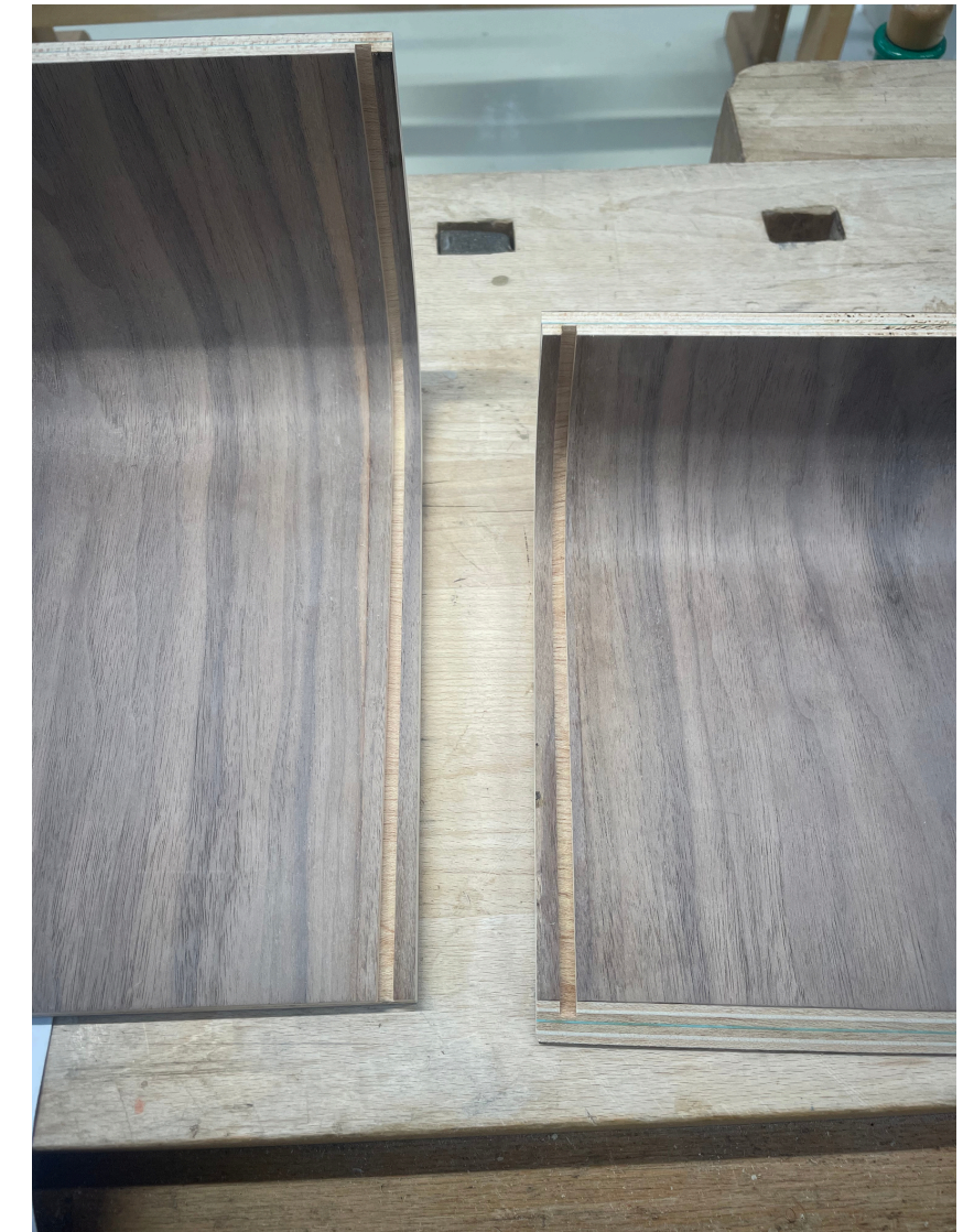
résultat de la rainure (fente permettant de venir imbriquer une pièce).
