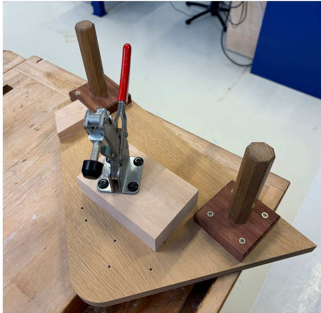
Montage d'usinage pour les pièces de bois massif qui deviendront le gabarit de collage.
